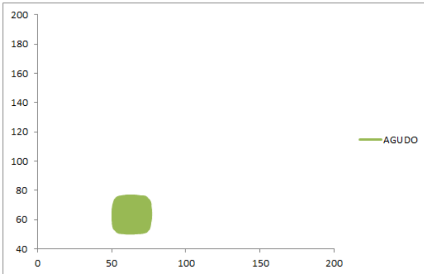
Figura 2. Atractor de una dinámica crónica o en evolución hacia la enfermedad aguda en 18 horas, con espacios de ocupación de K_p=184 , K_g=49 y DF=1,90885 (No. 33 de la tabla 2).
